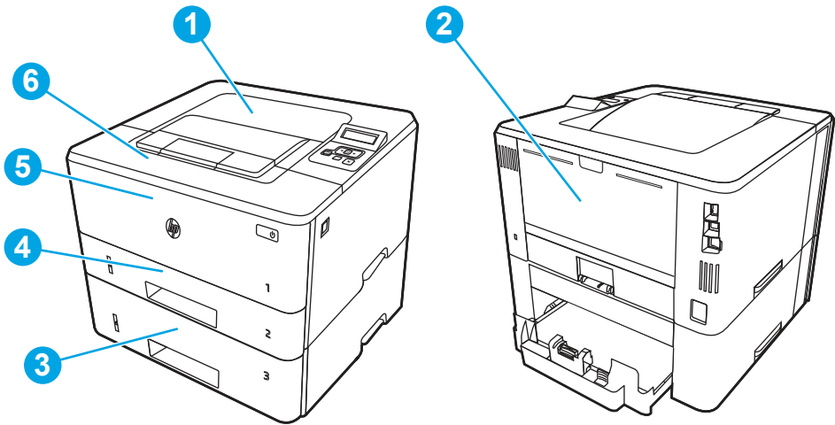
Figura 6-7 Locais de atolamento de papel
