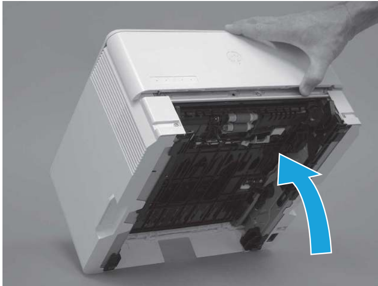
Figura 6-13 Inclinar a impressora para trás
