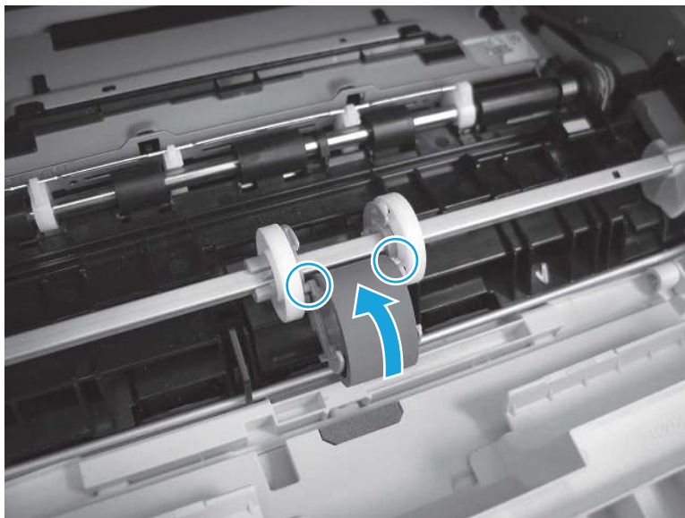
Figura 6-11 Instalar o cilindro
