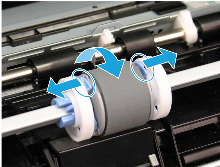
Figura 6-8 Liberar o cilindro
