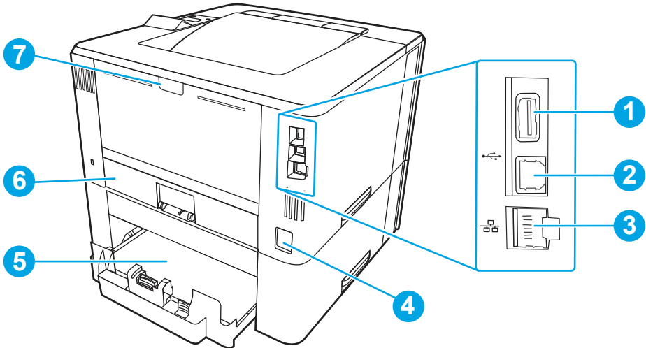
Figura 1-7 Vista traseira da impressora
